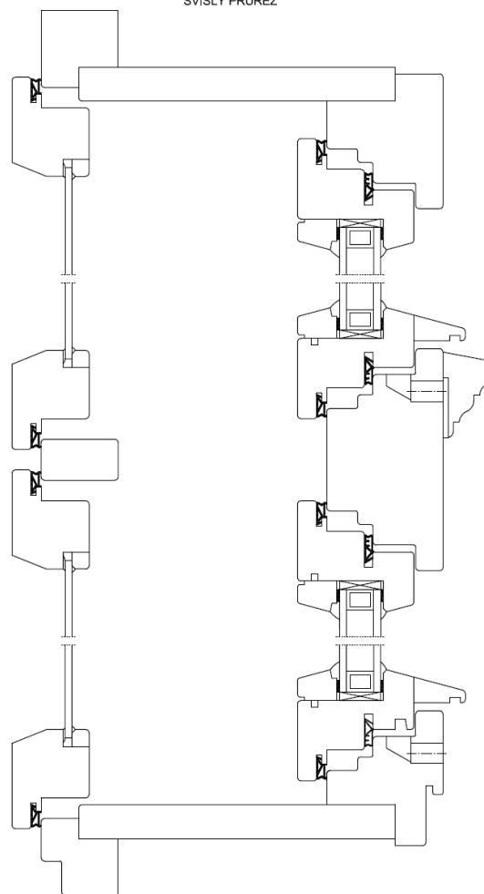
ŠPALETOVÁ OKNA SVISLÝ PRŮZEC
