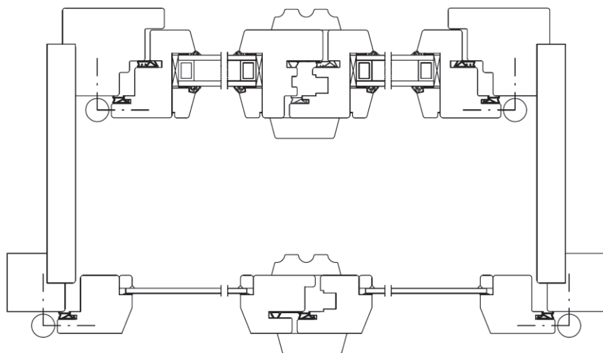
ŠPALETOVÁ OKNA VODOROVNÝ PRŮZEC
